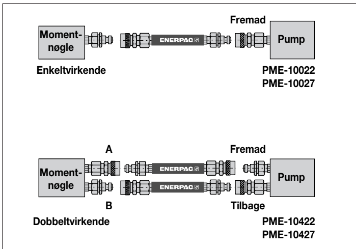
Figur 4 - Koblingsdiagram
