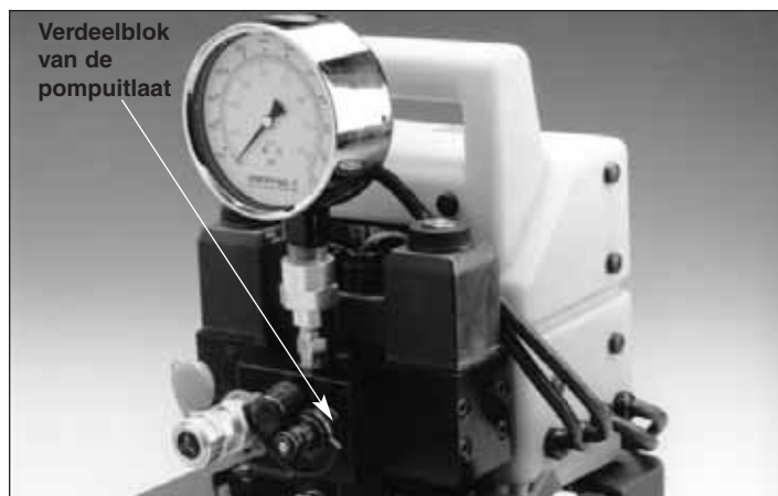
Afbeelding 3, Verdeelblok van de pomputlaat
