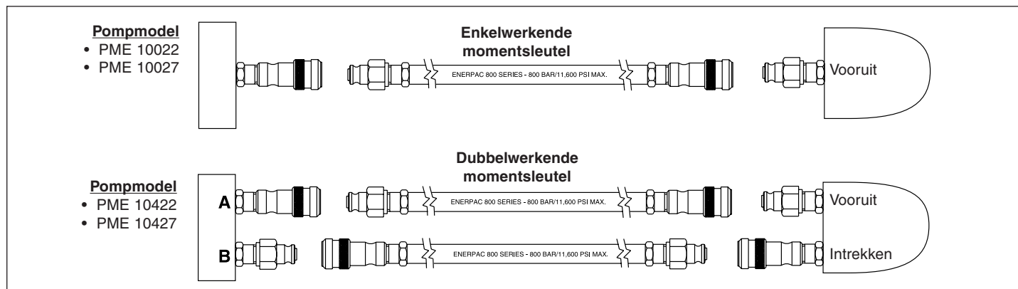
Afbeelding 4 – Aansluitschema
