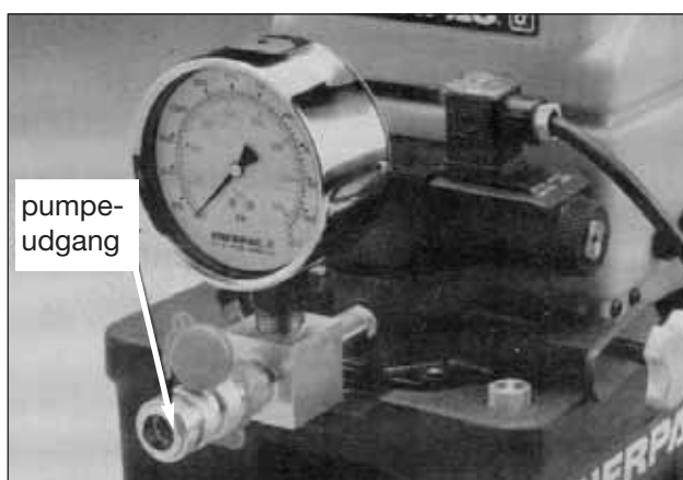
Figur 2 - Pumpeudgang
