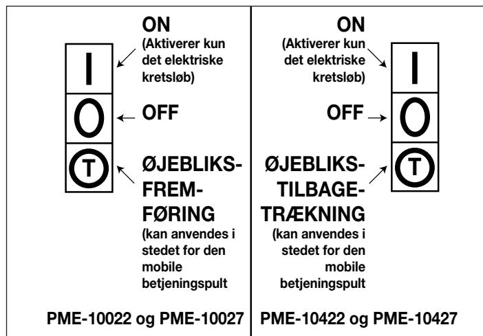
Figur 5 - Pumpekontaktens positioner
