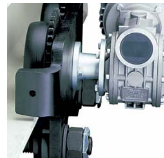
Radbruchstütze mit Möglichkeit zum Pufferbau
