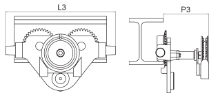
Modell HTG mit schwenkbarer Handkettenführung und Anfahrpuffern 500 - 5.000 kg
