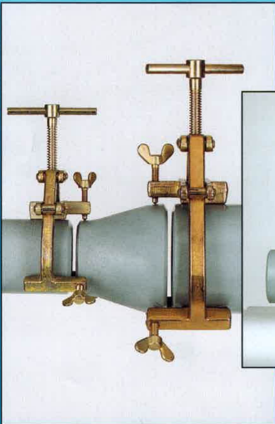
◀ Rohr - Reduzierung - Rohr Pipe - Pipe Reducer - Pipe
