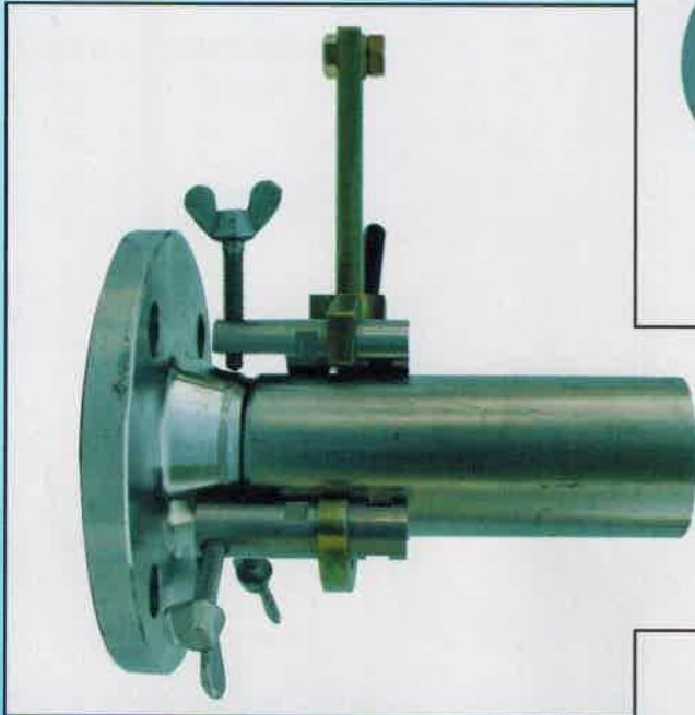
▲ Flansch - Rohr Flange - Pipe
