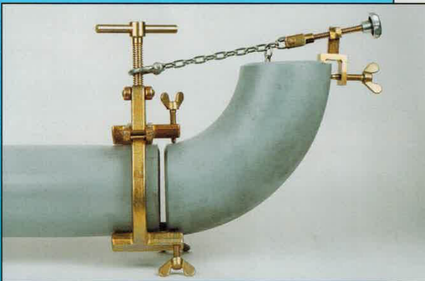
Rohr - Rohrbogen mit Haltevorrichtung ▼ Pipe - Tube Turn with Holding Device
