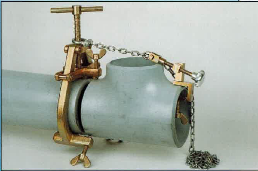
▲ Rohr - T-Stück mit Haltevorrichtung Pipe - Tee with Holding Device
