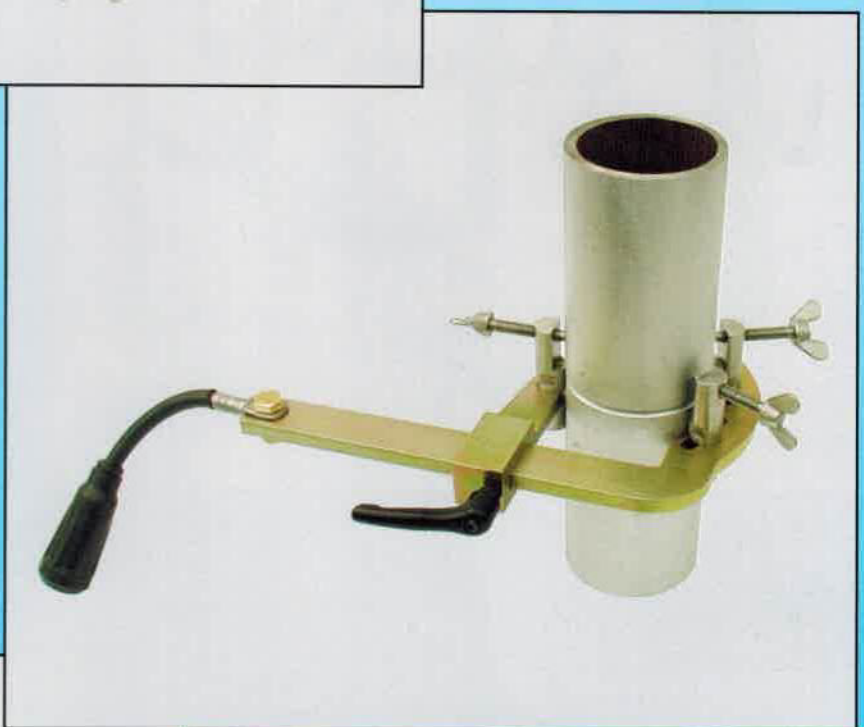
▲ Rohr – Rohr, mit Masse-Anschluss Pipe – Pipe, Earth Clamp
