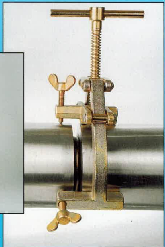
Rohr - Rohr ▶ Pipe - Pipe
