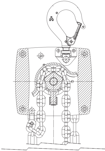
Yalelift 0,5 - 3t
