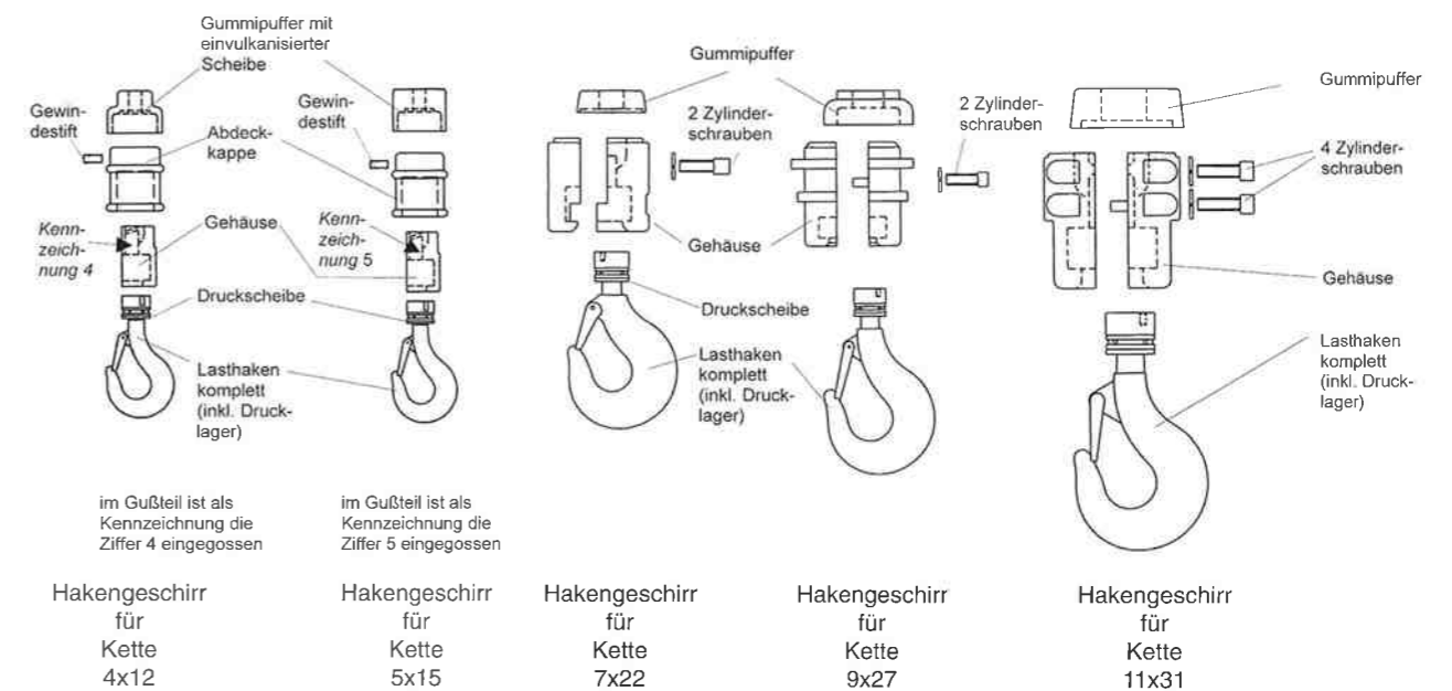
Bild 4: Aufbau der Hakengeschrirre
