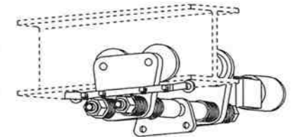
Bild 24: Gegenrollen für Massenausgleich an Fahrwerken
