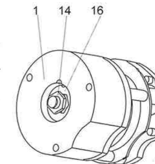
Bild 30: Einstellmutter für Kupplungskraft
