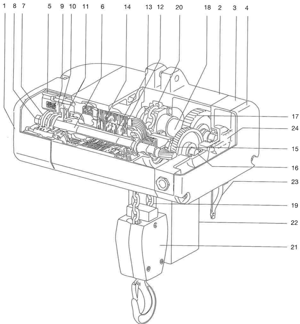
Bild 2: Schnittbild
