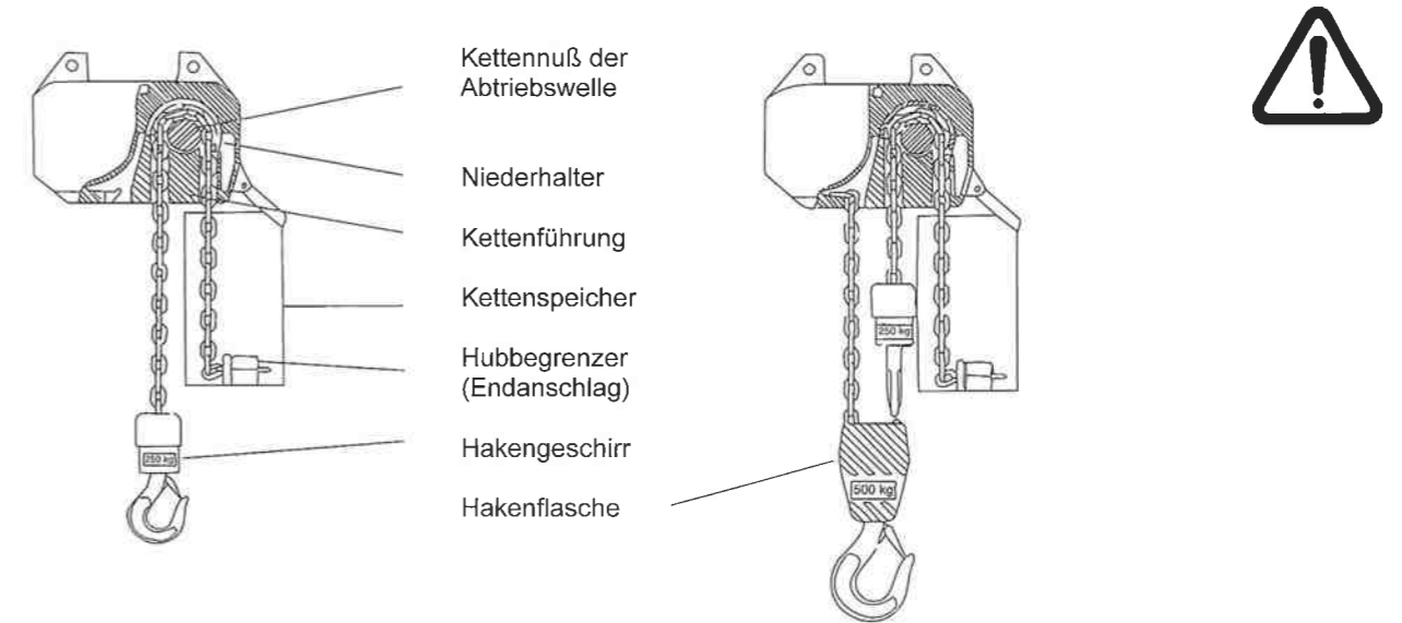
Bild 3: 3.1 einsträngige Ausführung
