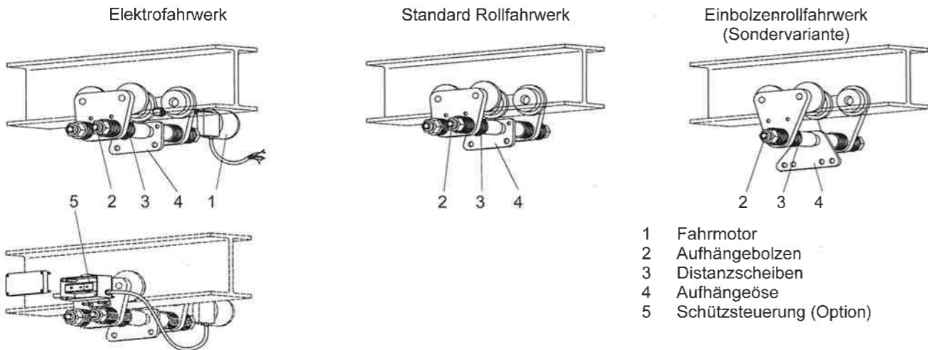
Bild 21: Fahrwerk
