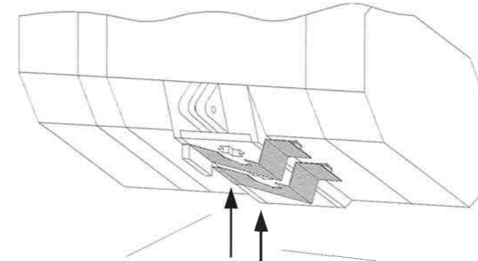
Bild 20: zusätzliche elektrische Endschalter bei 24 V Kleinspannung
