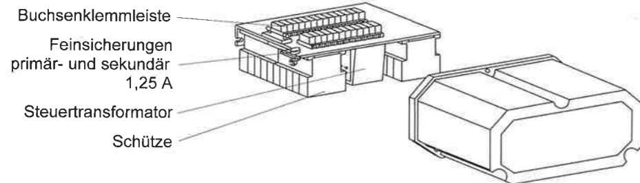
Bild 19: Kleinspannungssteuerung
