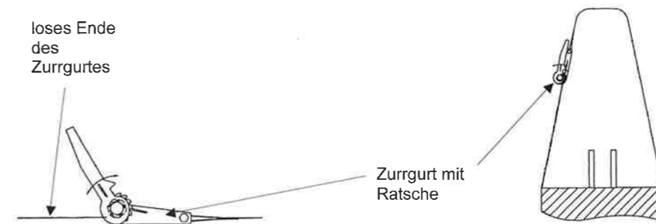
Bild 13: Schema des Einfädelns und des Spannsens des Zurr gurt es in der Ratsche
