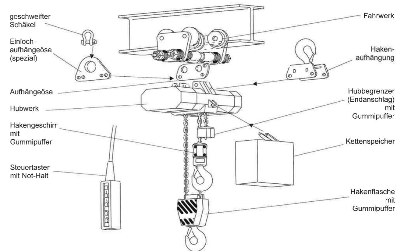
Bild 1: Komplettierungsmöglichkeiten
