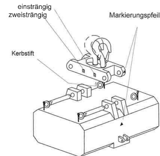
Bild 8: Aufhängung mit Hakenaufhängung der Bauformen 2-9.1
