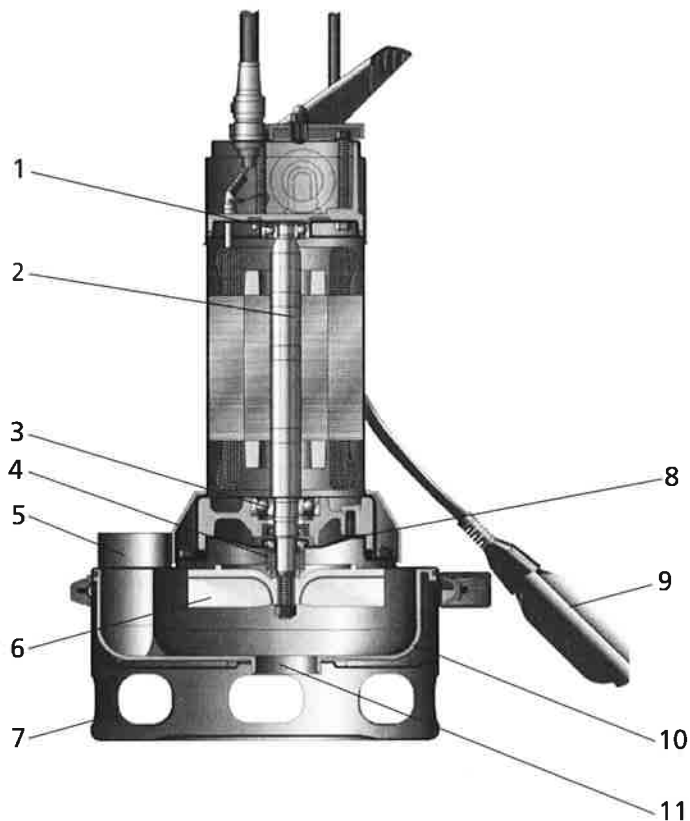
Abb. 2: Schnittbild
