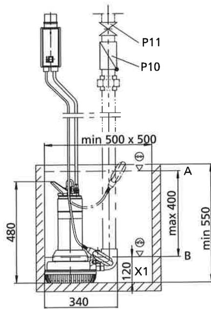
Abb. 11: Maßzeichnung Ama-Drainer 522/11 ohne Kühlmantel
