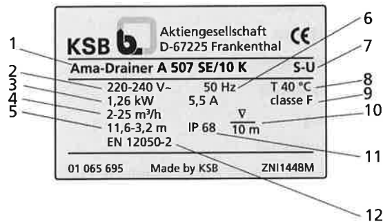
Abb. 1: Typenschild (Beispiel)
