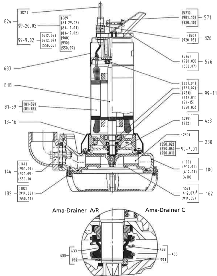
Abb. 7: Gesamtzeichnung Ama-Drainer 522/11
