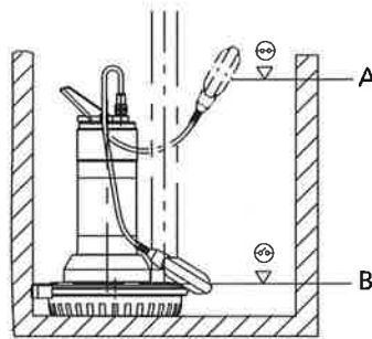
Abb. 4: Ein- / Ausschaltpunkt
