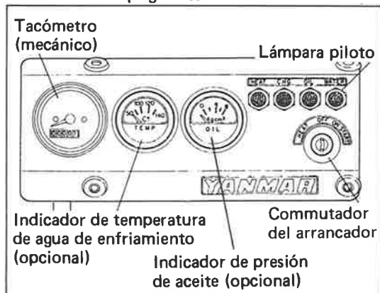
Panel de serie Yanmar
