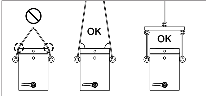
Abbildung 3: Hubeinrichtung (typisch)
