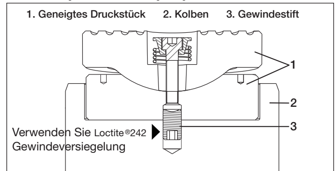
Abbildung 4, Zubehör der CATS-Serie, geneigtes Druckstück (typisch)
