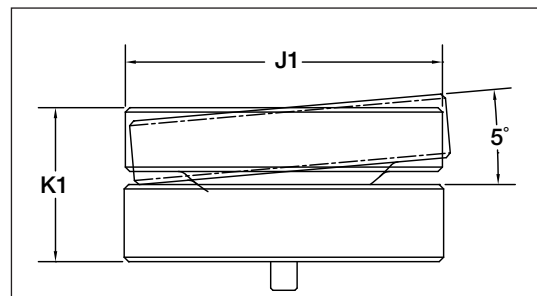
Abbildung 7, Abmessungen - HCL-Serie
