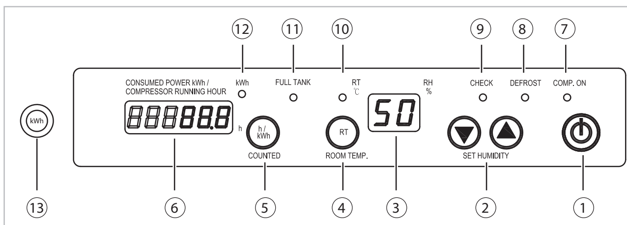
Abb. 8: Bedienungstableau
