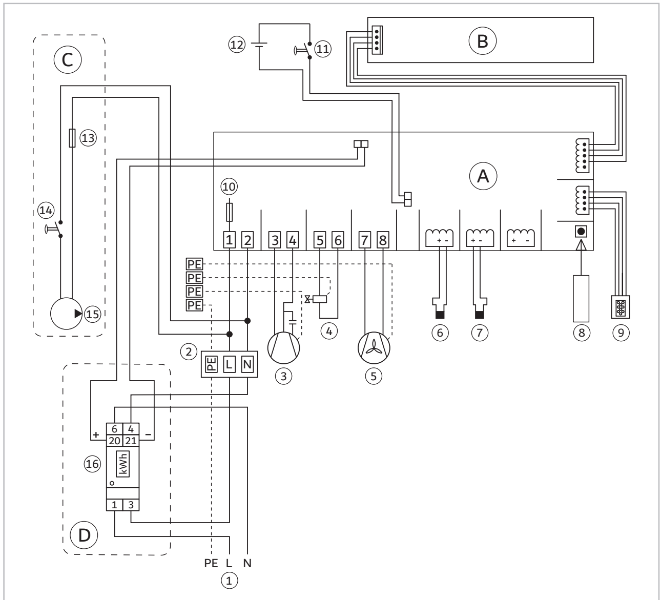
Abb. 7: Elektrisches Anschlussschema
