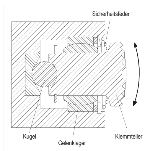
Funktionsskizze Palle
