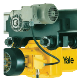
Direktangebundenes Fahrwerk mit elektrischem Antrieb, auch Roll- und Haspelfahrwerke lieferbar.
