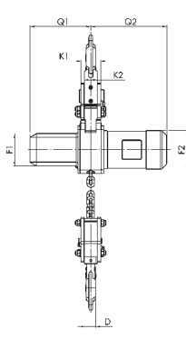
Yale CPEF mit Traghaken, einsträngig 1.600 - 3.000 kg
