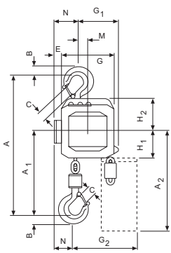
Yale CPEF mit Traghaken, einsträngig 1.600 - 3.000 kg
