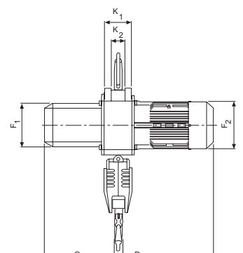
Yale CPEF mit Traghaken, zweisträngig 3.200 - 5.000 kg
