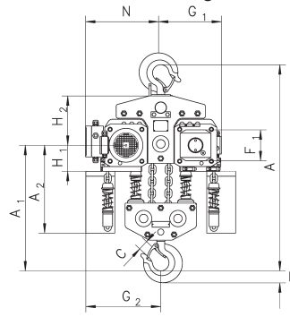
Yale CPEF 100-2 mit Traghaken 10.000 kg
