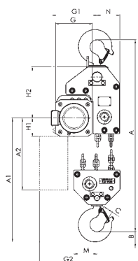
Yale CPEF 75-1,6 mit Traghaken 7.500 kg
