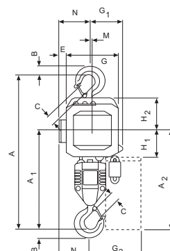
Yale CPEF mit Traghaken, zweisträngig 3.200 - 5.000 kg
