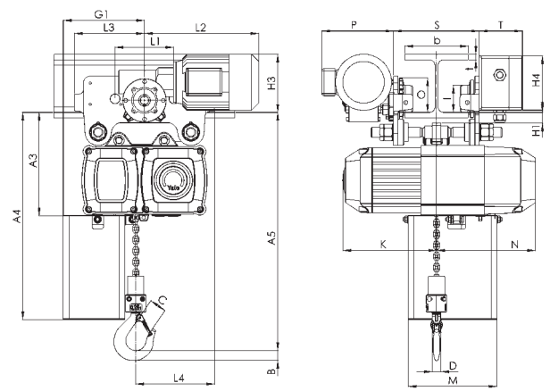
Yale CPV/CPVF Festverbindung mit Elektrofahrwerk
