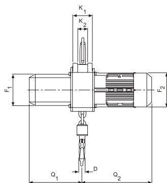
Yale CPEF mit Traghaken, einsträngig 1.600 - 3.000 kg
