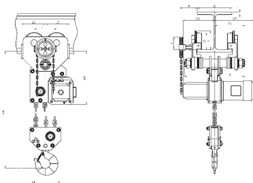
Yale CPEF 75-1,6 mit Haspel- oder Elektrofahrwerk 7.500 kg
