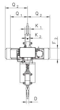
Yale CPEF mit Traghaken, zweisträngig 3.200 - 5.000 kg
