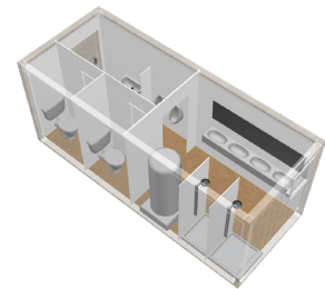
SANITÄR-CONTAINER
