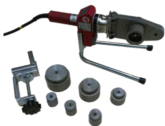
MUFFENSCHWEISSGERÄT
