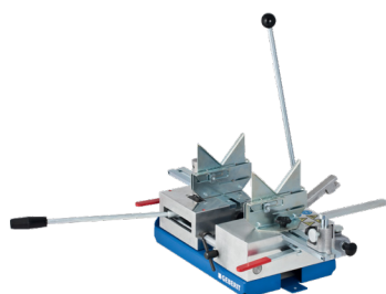
STUMPSCHWEISSGERÄT
