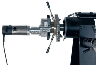
ROHRANFASGERÄTE INNENSPANNER
